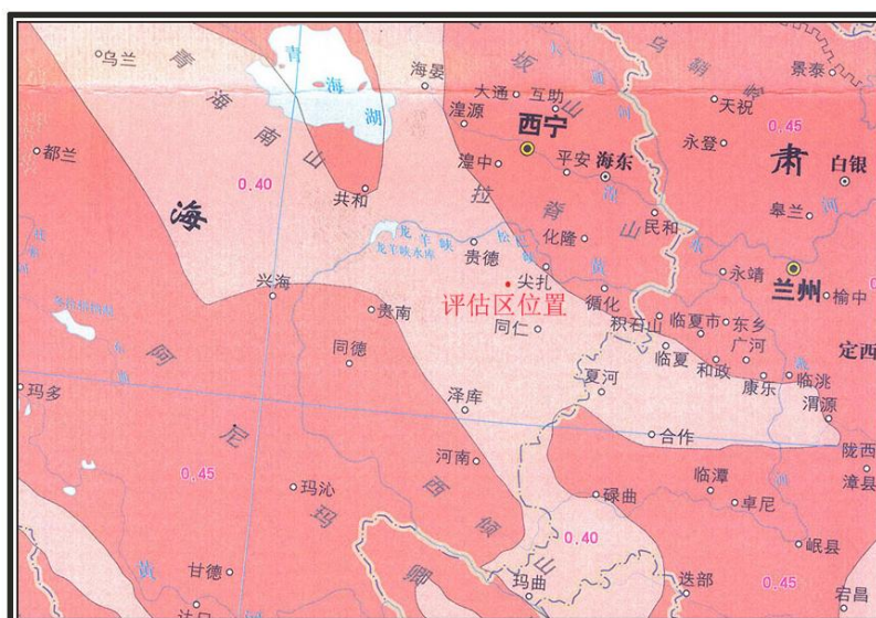
图 2-3 项目区中国地震动峰值加速度区划图
